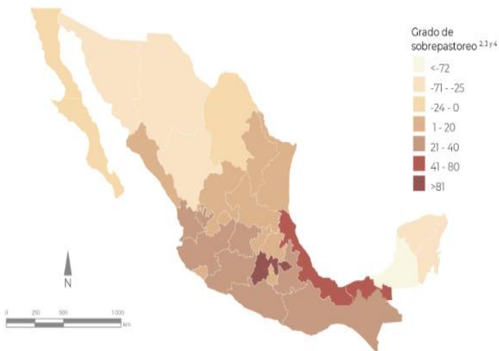
Mapa 2.13 Grado de sobrepastoreo por entidad federativa, 2016 1
