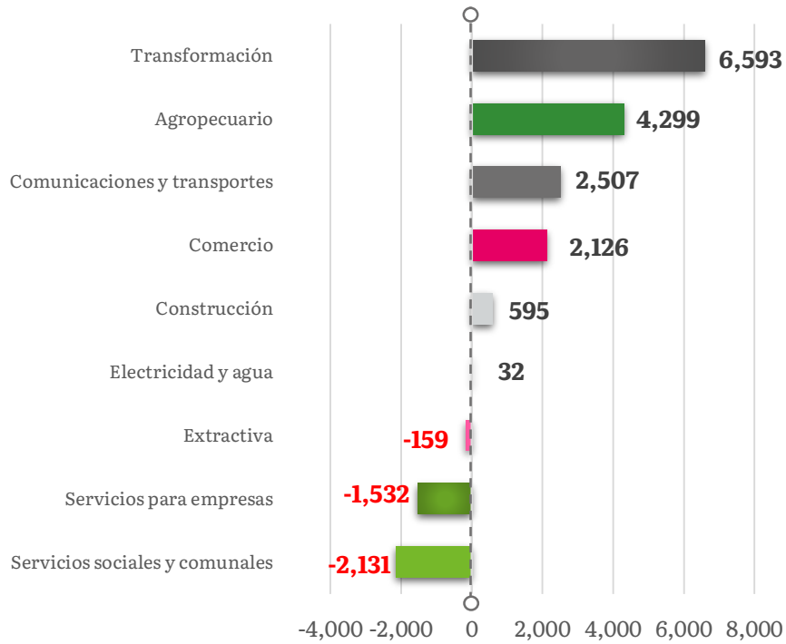
Gráfico No.5 San Luis Potosí Trabajadores asegurados del IMSS, según actividad económica Mayo 2021 - Mayo 2022 (Variación absoluta)
