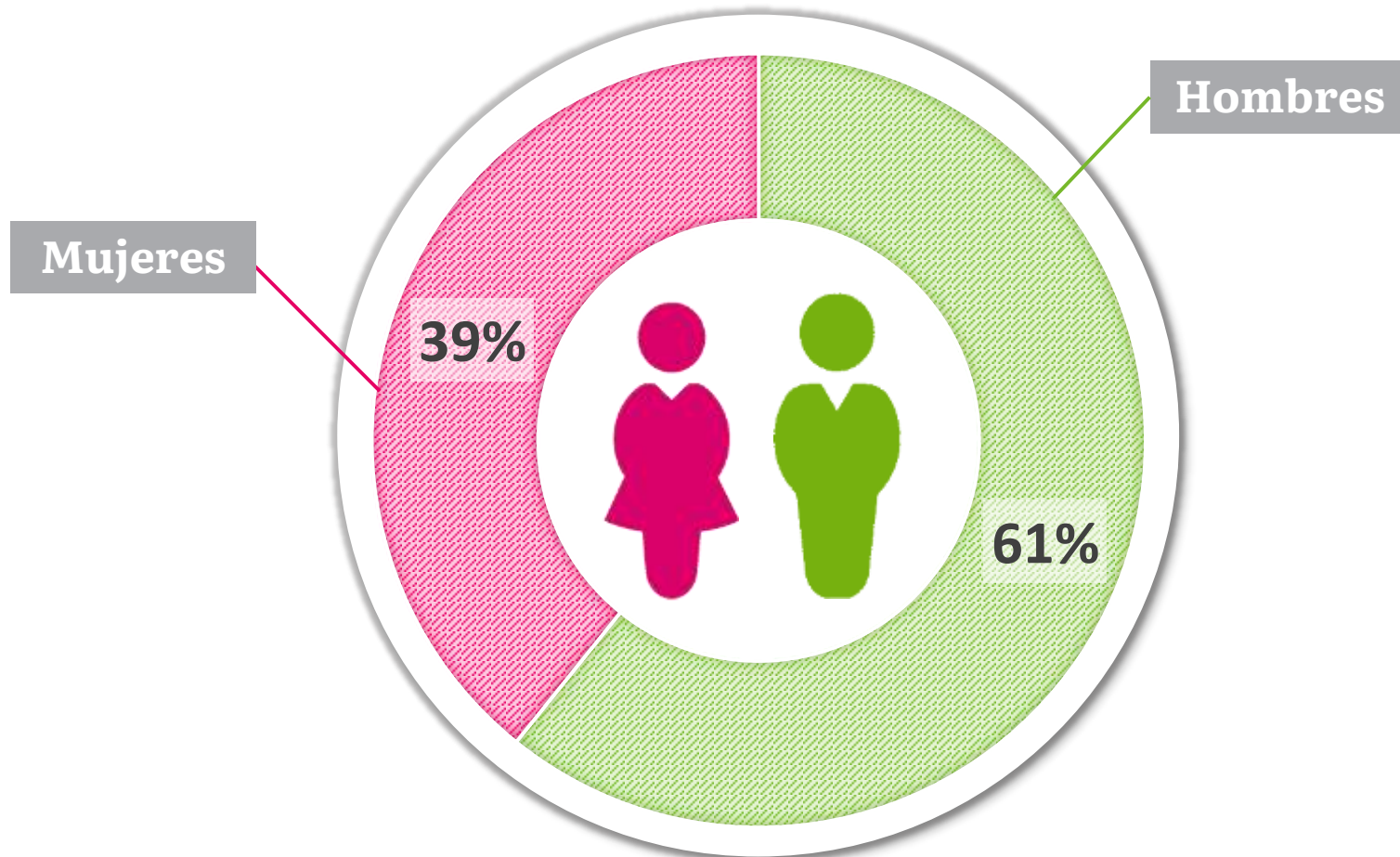
Gráfico No.3 San Luis Potosí Trabajadores asegurados en el IMSS, según sexo Mayo 2022 (Participación)
