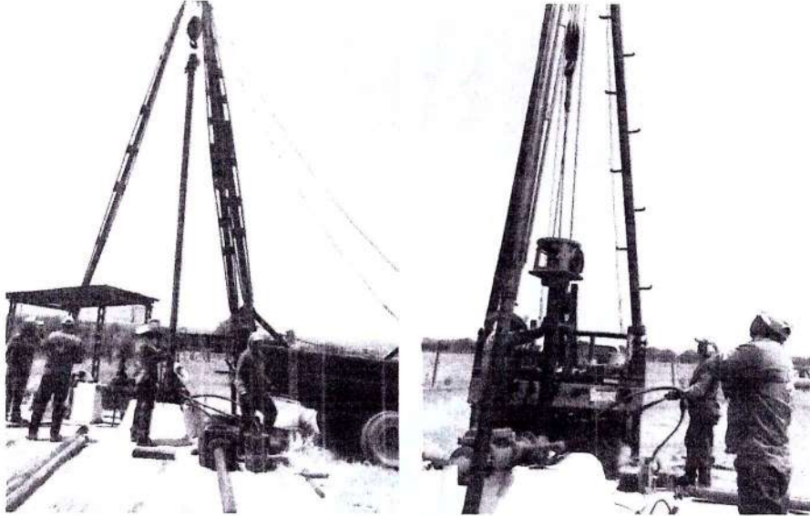
Fotografías de la instalación de la tubería en la columna del pozo
