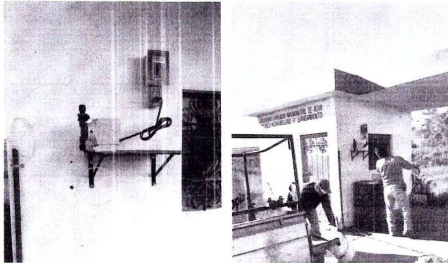
Fotografías de la instalación de la tubería en la columna del pozo
